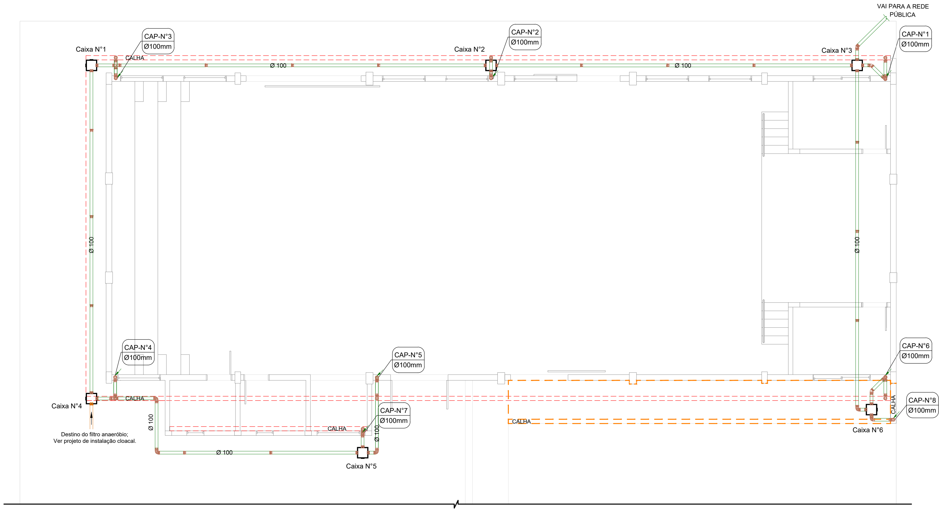
INSTALAÇÃO PLUVIAL Escala: 1/75
